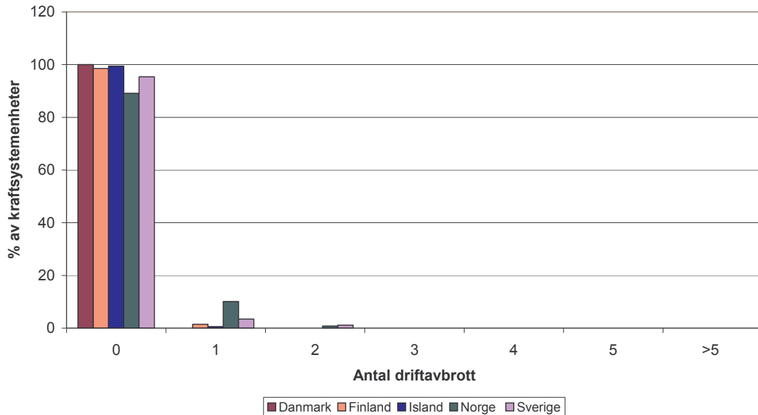
Figur 6.2. Driftavbrott för samlingsskena för alla länder under 2004
