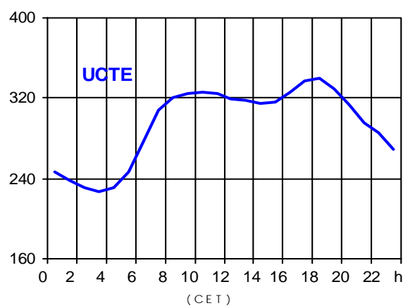
17.12.2003 ( in GW )
