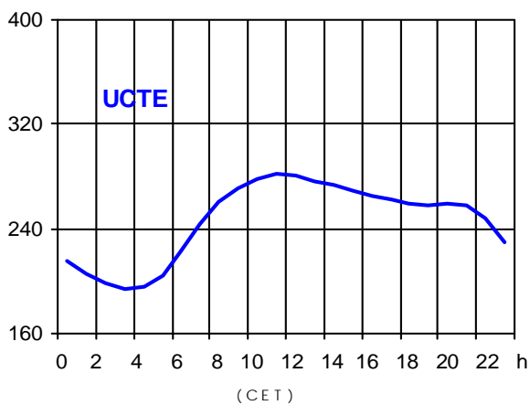
17.09.2003 ( in GW )
