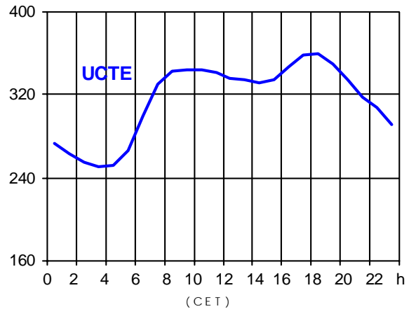
17.12.2003 ( in GW )
