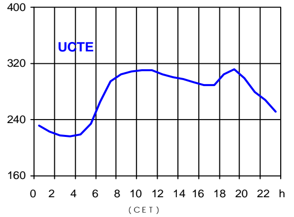
19.11.2003 ( in GW )
