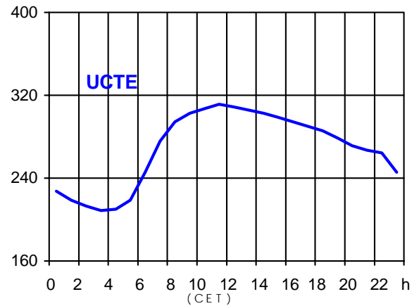
18.06.2003 ( in GW )
