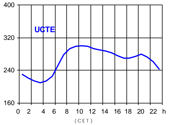
21.05.2003 ( in GW )
