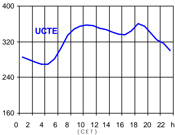
19.03.2003 ( in GW )
