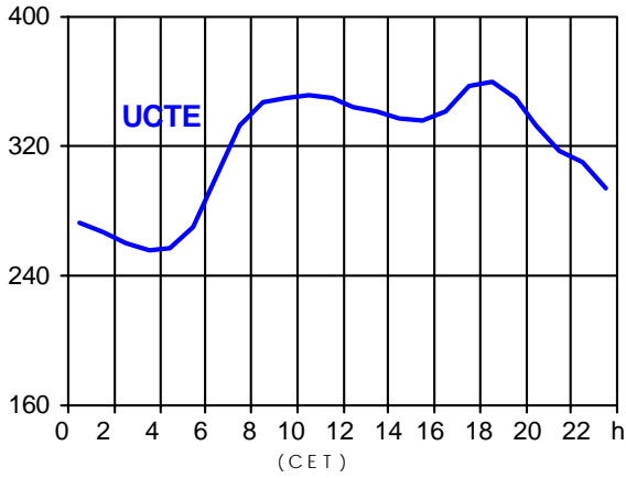
19.02.2003 ( in GW )
