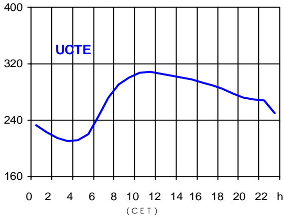
20.08.2003 ( in GW )
