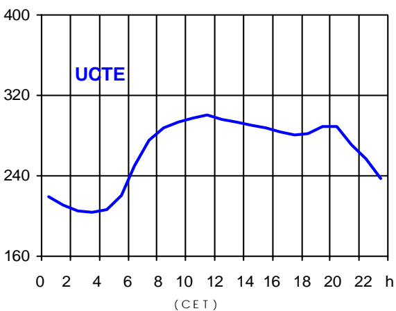
17.09.2003 ( in GW )
