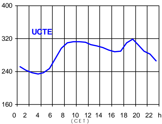
19.03.2003 ( in GW )
